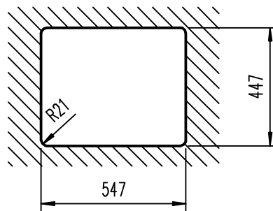
Ausschnitt flächenbündig 1:20
